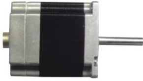
CWN-B0070 左剪刀电机 OMNIplus 800 BE305382
