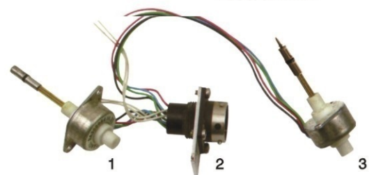
CWN-B0063 主喷电磁阀转子 BA300086 (1)
