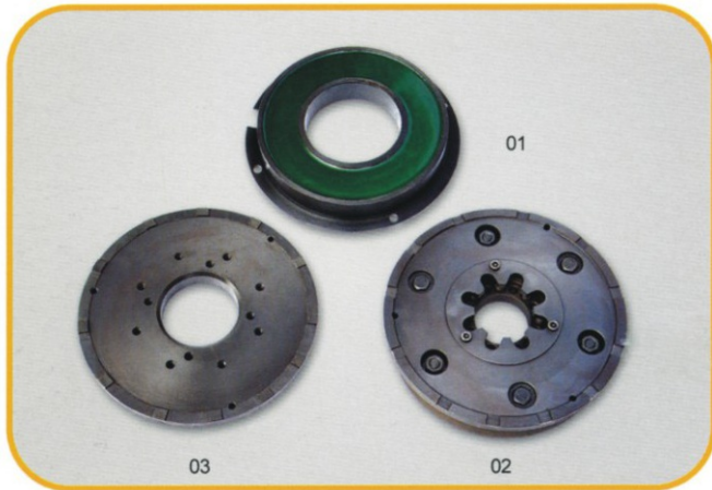
01-寻纬线圈 02-寻纬齿盘 03-侧齿盘
