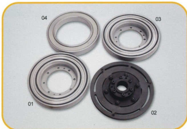
01-制动器线圈 02-衔铁 03-摩擦轮 04-离合器线圈
