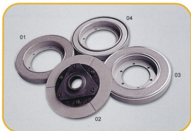
01-制动器线圈 02-衔铁 03-转动轮 04-离合器线圈
