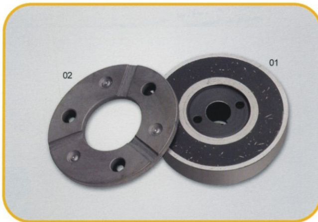
01-离合器线圈 02-衔铁
