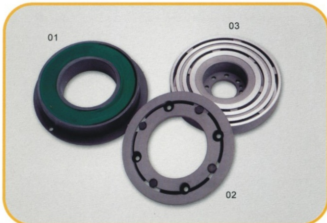
01-离合器线圈 02-衔铁 03-转动轮
