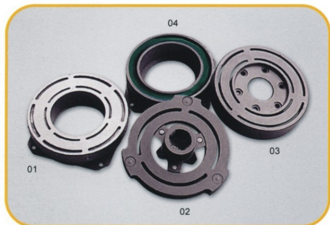
01-制动器线圈 02-衔铁 03-转动轮 04-离合器线圈
