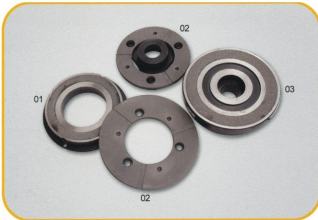
01-制动器线圈 02-衔铁 03-离合器线圈
