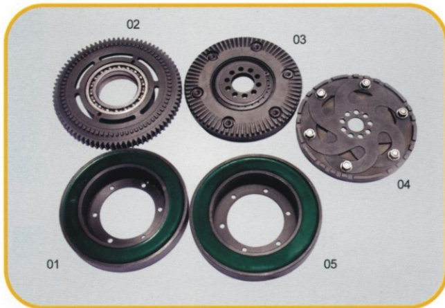
01-慢速线圈 02-慢速齿轮 03-双面齿盘 04-寻纬齿盘 05-寻纬线圈
