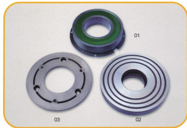
01-慢速线圈 02-慢速转动轮 03-慢速衔铁
